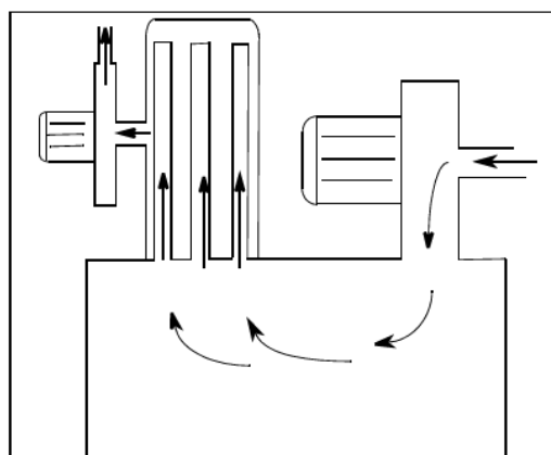
Billedet viser flowet mellem hammermølle, blander og filter. PRESIDENT leverer støvfrit anlæg med en kapacitet op til 3500 kg/t.
