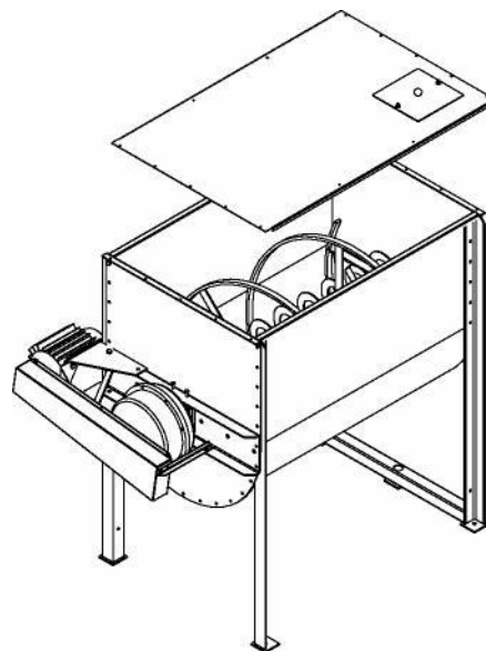
PRESIDENT Horisontalblander PHB8 – standard-udførelse
