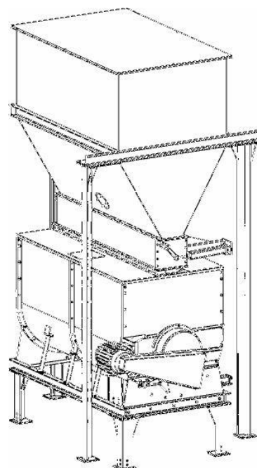
PRESIDENT horisontalblander PHB20 vist med forbeholder og spjældkasse
