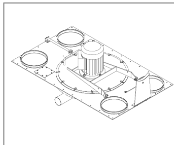
PRESIDENT hammermølle type HMS vandretliggende mølle.
