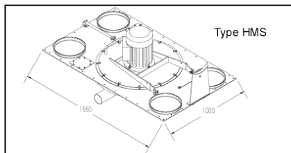
PRESIDENT hammermølle type HMS vandretliggende mølle.
